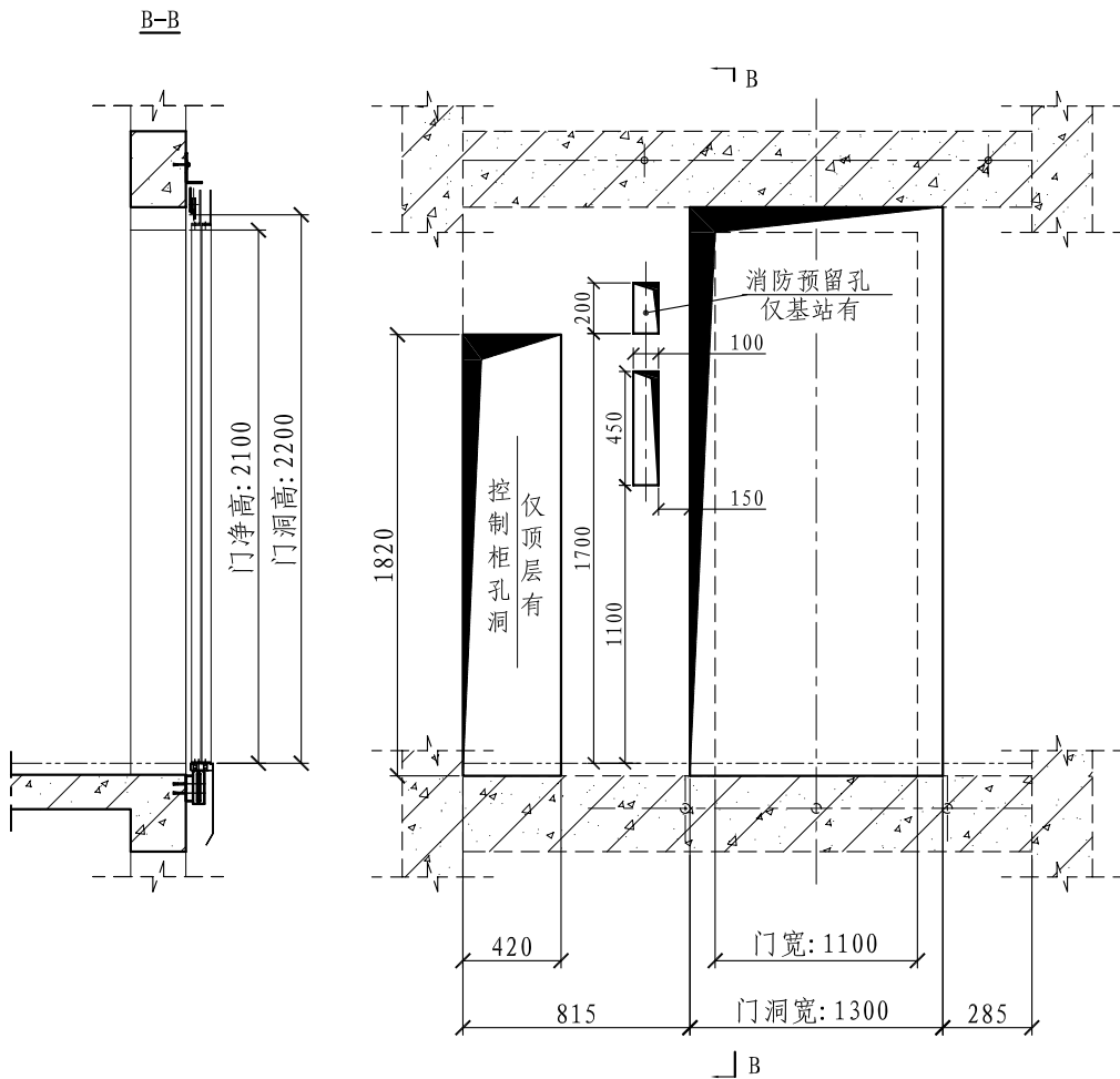
厅门预留孔图 井道宽度2400
