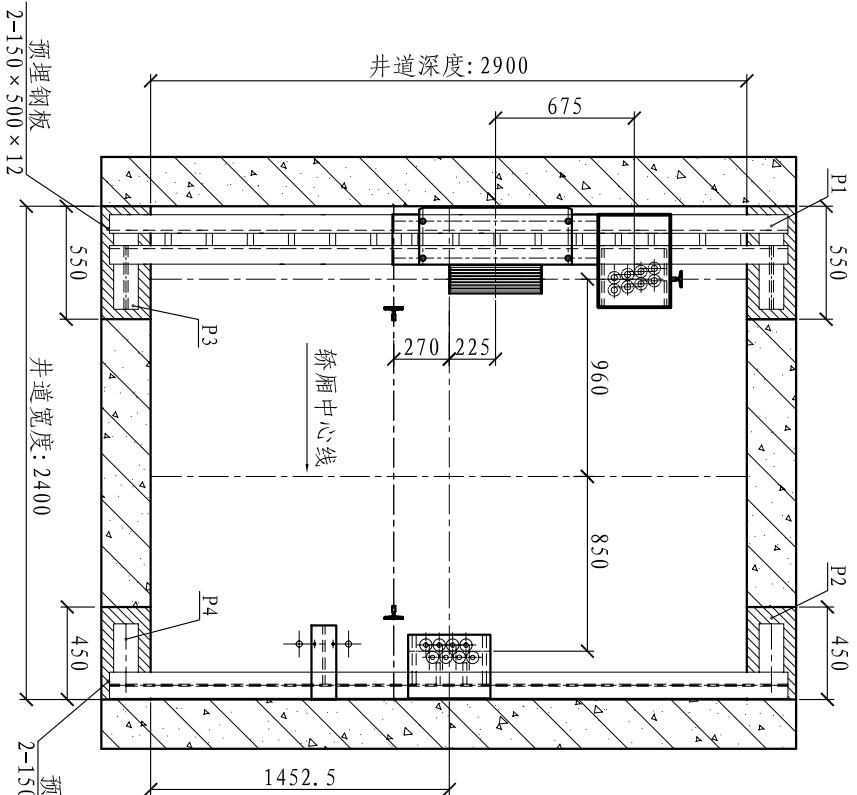
井道顶部承重梁布置图
