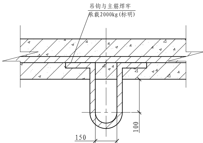
井道顶部维修吊钩 (供参考, 结构尺寸由土建设计定)
