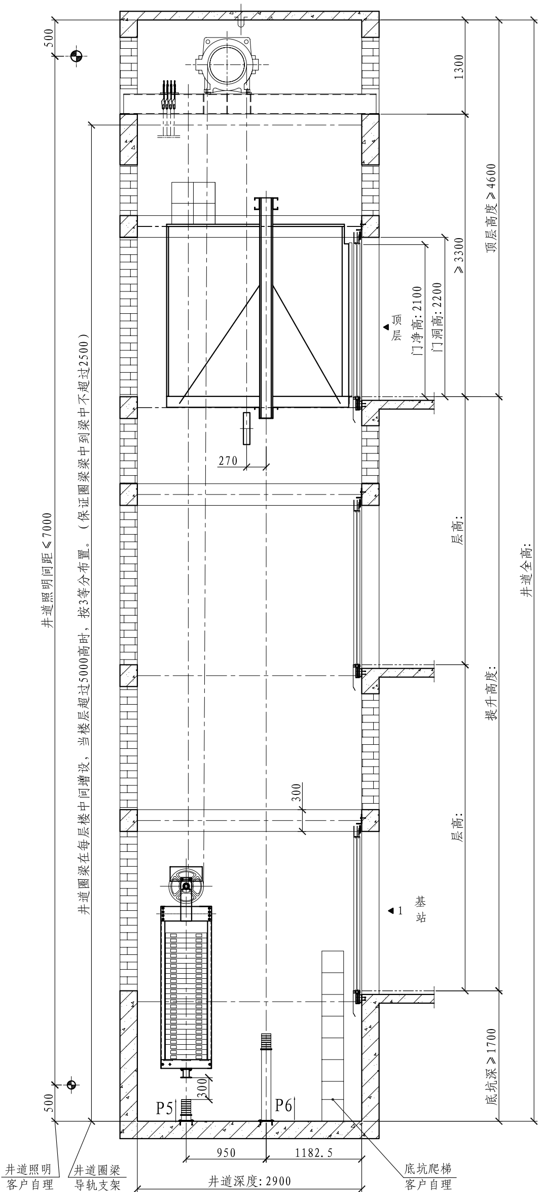
井道立面图 (共安装参考)
