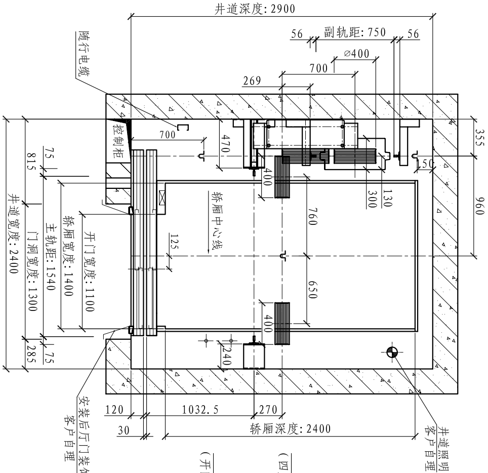
井道平面布置图
