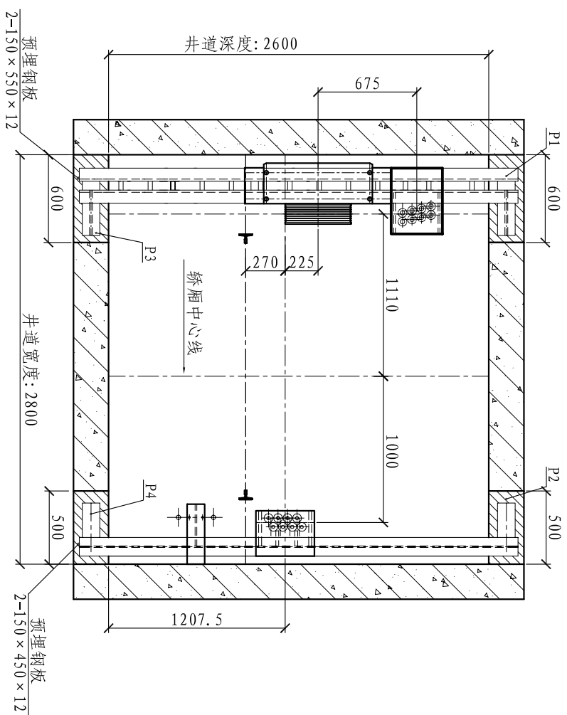
井道顶部承重梁布置图
